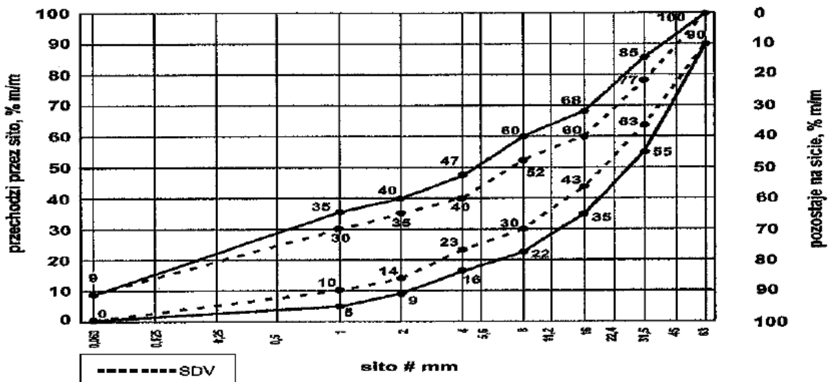
Rysunek 2. Krzywe graniczne uziarnienia mieszanki kruszywa niezwiązanego 0/45 mm do warstw podbudowy zasadniczej
