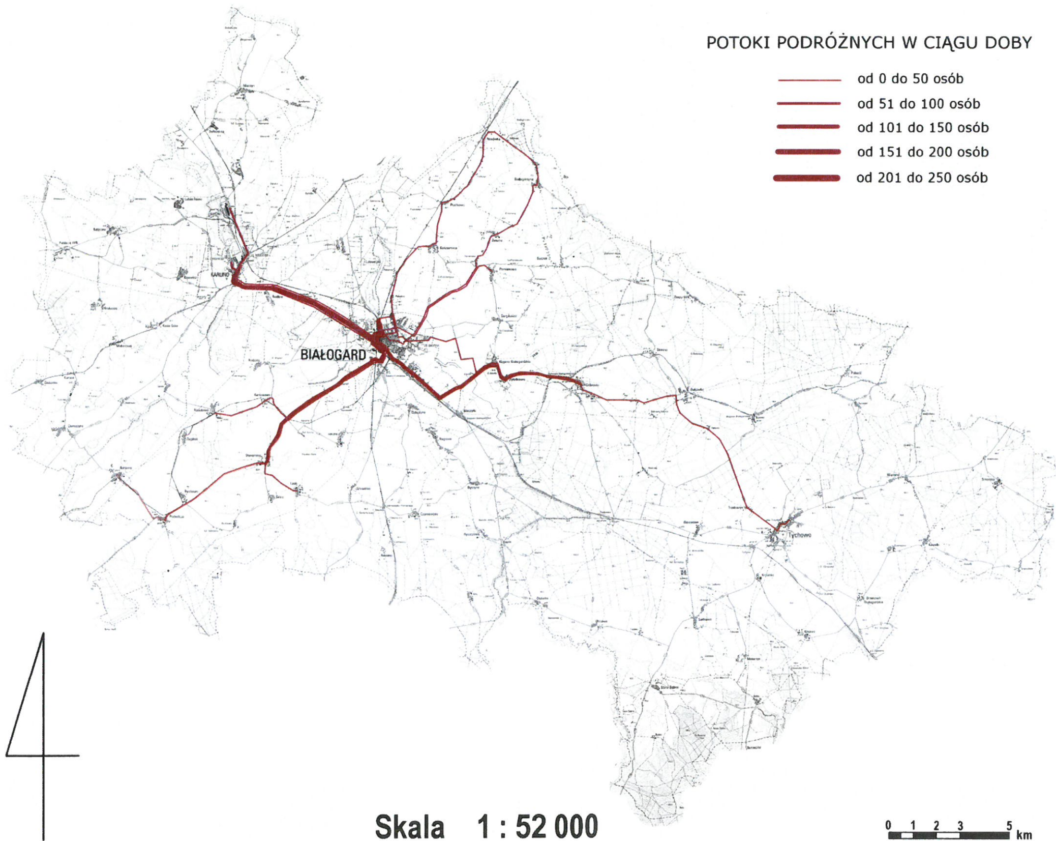
Rys. 9. Średnie dobowe natężenie podróży na poszczególnych trasach (potoki podróży)
